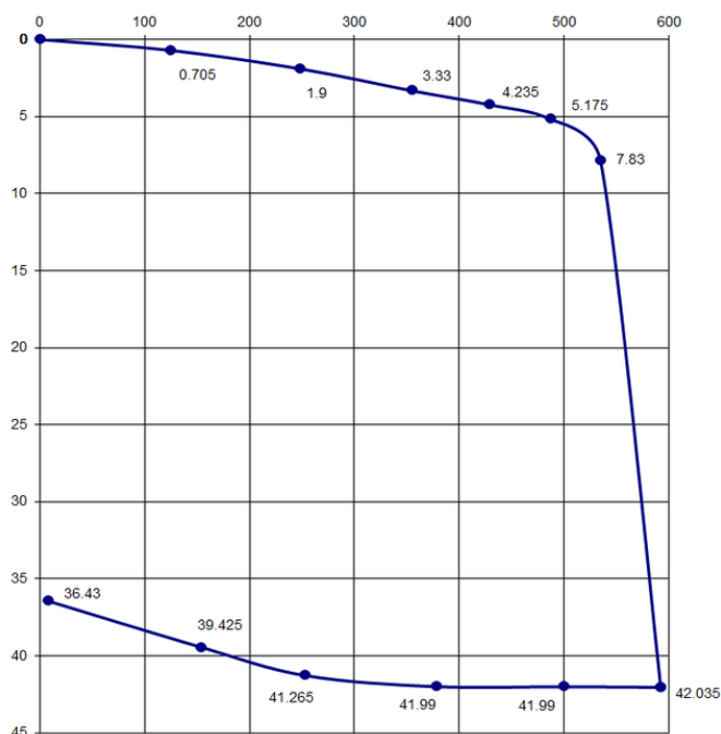
Рис.2. Використання випробування палей для ідентифікації параметрів ґрунту Fig.2. Use piling tests to identify soil parameters
